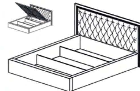
Богера 3 Ліжко (каркас)/ Bed (frame) 160 187/106/215 180 207/106/215 шир./вис./довж./W/H/L
