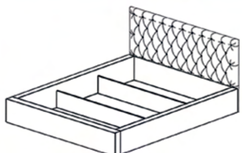
Богера 2 Ліжко (каркас)/ Bed (frame) 160 178/109/215 180 198/109/215 шир./вис./довж./W/H/L
